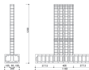
図1 試験体配筋図
