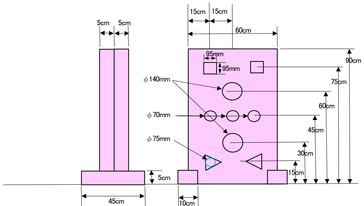
断面図
